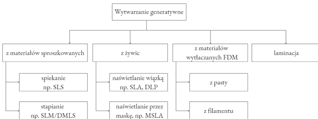
Rys. 34. Podział technologii generatywnych [26]
