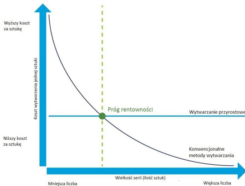
Rys. 38. Krzywa opłacalności druku 3D w porównaniu do technologii konwencjonalnych [15]
