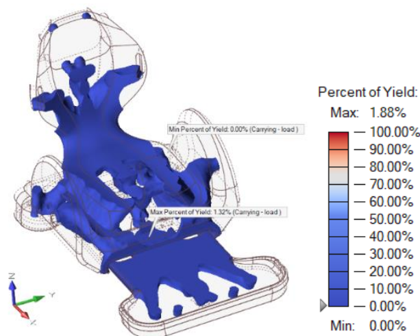
Rys. 122. Uplastycznienie materiału
