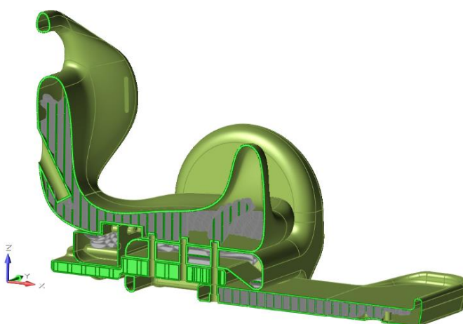
Rys. 128. Przekrój modelu złożenia z siatką typu grid o gęstości 20% wypełniającą strukturą zoptymalizowaną topologicznie
