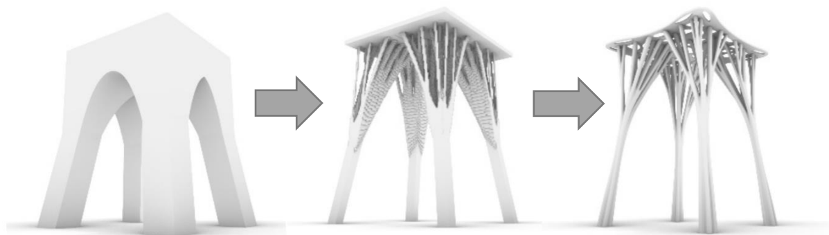
Rys. 23. Kolejne etapy optymalizacji konstrukcji pawilonu X-Form 1.0 [5]
