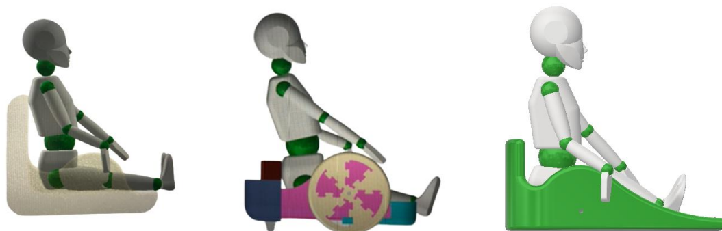
Rys. 44. Wirtualne testowanie ergonomii i sprawdzenie odpowiednich wymiarów dla różnych koncepcji pojazdu
