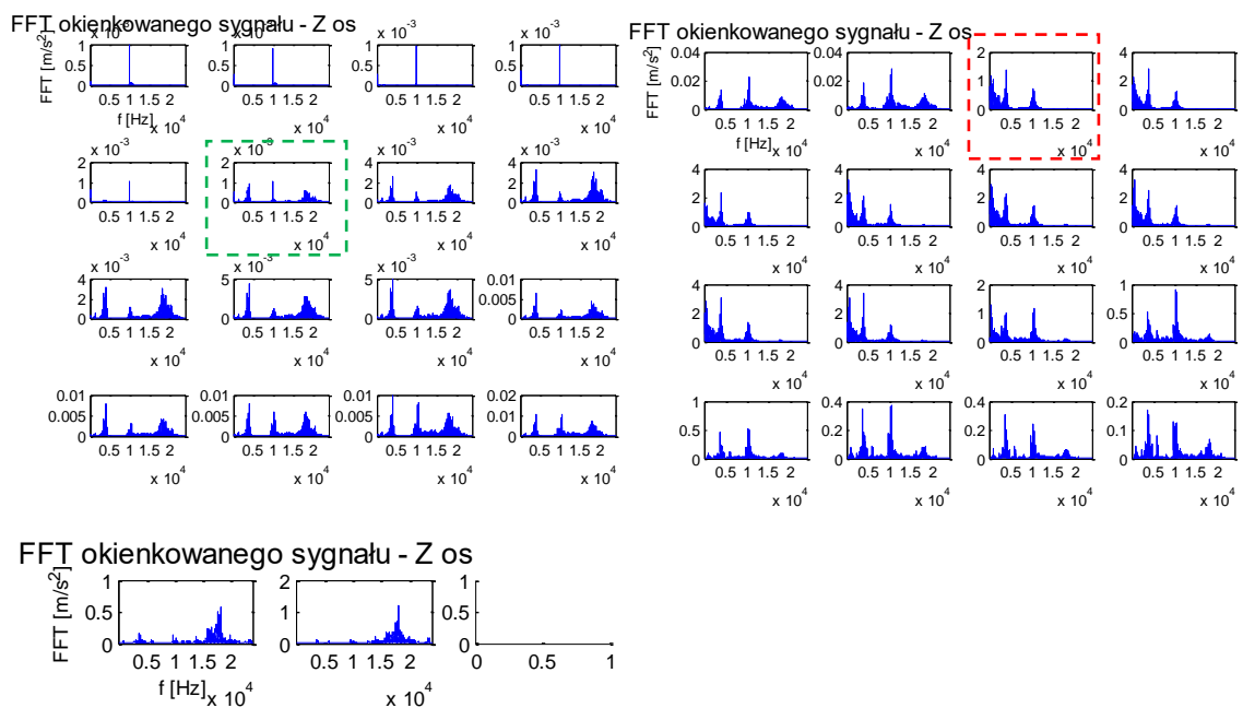
Rys. 109 Widma drgań w kolejnych oknach sygnału, okna 1-35 (oś Z), dla składu: pociąg towarowy – 18 węglarek, prędkość 40 km/h.
