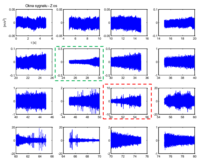
Rys. 91 5-sekundowe okna sygnału dla osi Z.
