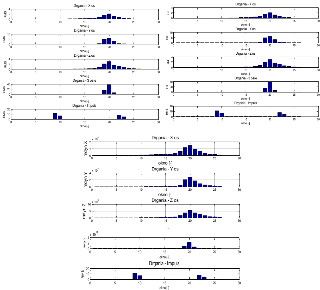
Rys. 88 Zestawienie rozkładów wybranych miar dla 3-sekundowych okien.
