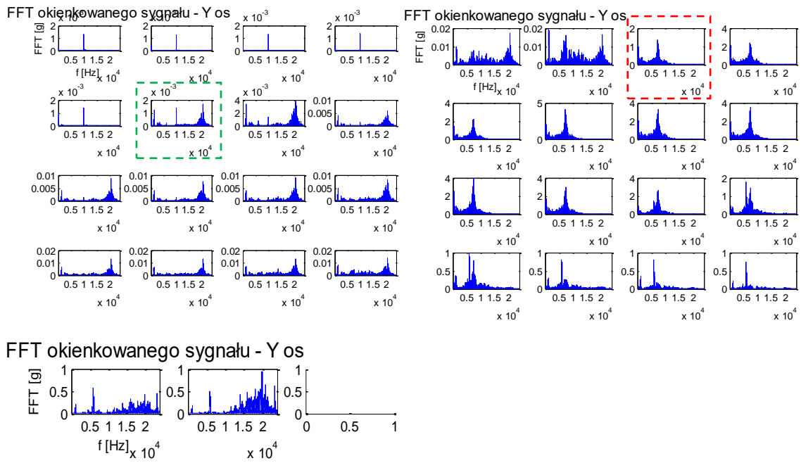
Rys. 108 Widma drgań w kolejnych oknach sygnału, okna 1-35 (oś Y), dla składu: pociąg towarowy – 18 węglarek, prędkość 40 km/h.
