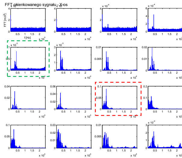
Rys. 92 Widma 5-sekundowych okien sygnału dla osi X.
