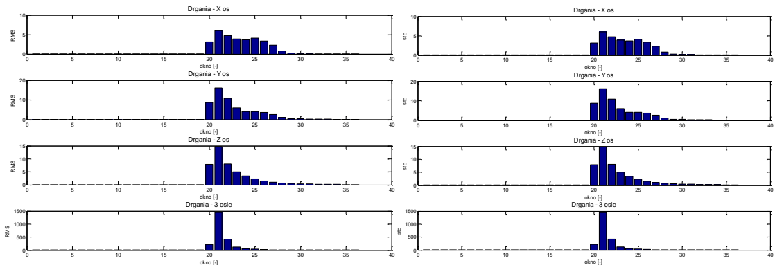
Rys. 130 Rozkład wartości skutecznej oraz rozkład wartości odchylenia standardowego drgań zarejestrowanych w 3 prostopadłych osiach, dla składu: pociąg osobowy ELF-2, prędkość przejazdu 38 km/h.
