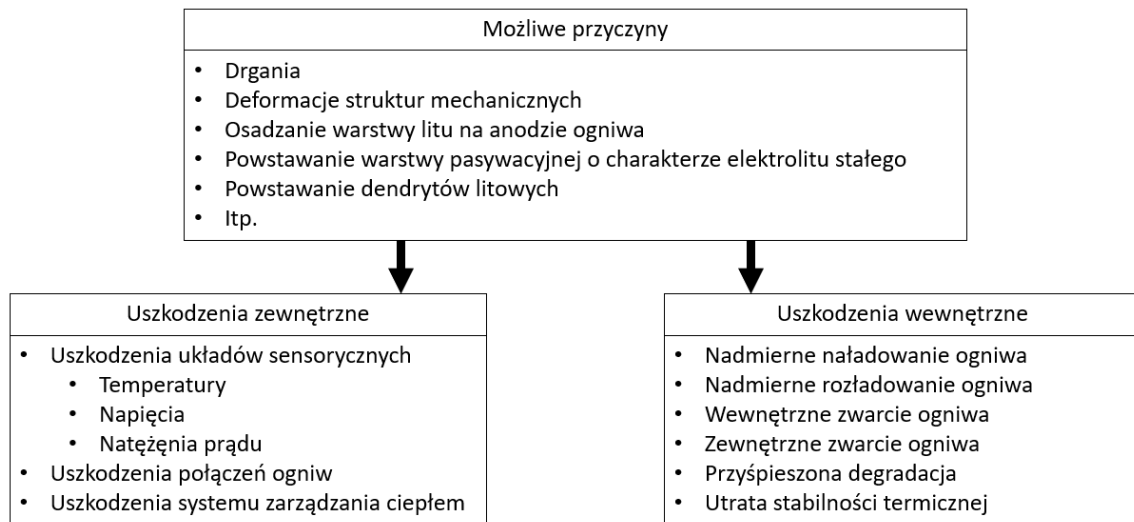
Rys. 2. Wewnętrzne i zewnętrzne uszkodzenia akumulatorów litowo-jonowych oraz ich przyczyny [4]
