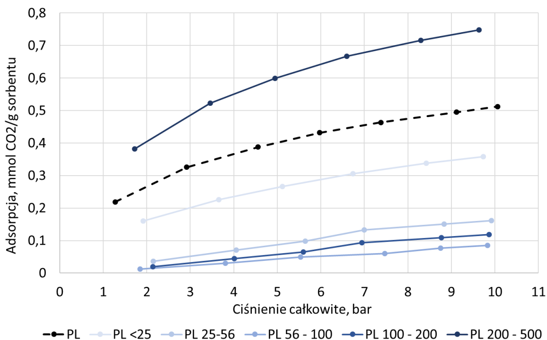
Rys. 9.5 Wykres adsorpcji CO 2 w funkcji ciśnienia bezwzględnego próbki PL z podziałem na frakcje ziarnowe
