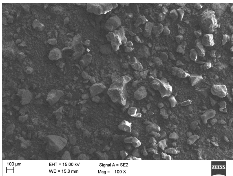
Rys. 9.2 Zdjęcia SEM (x100) próbek wykorzystywanych w badaniu: PL (góra) oraz PLZ (dół)
