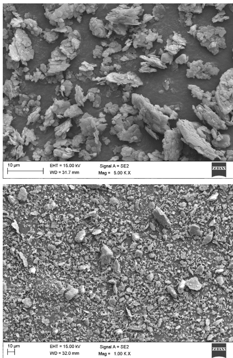
Rys. 4.2 Zdjęcia SEM kaolinu użytego w badaniach
