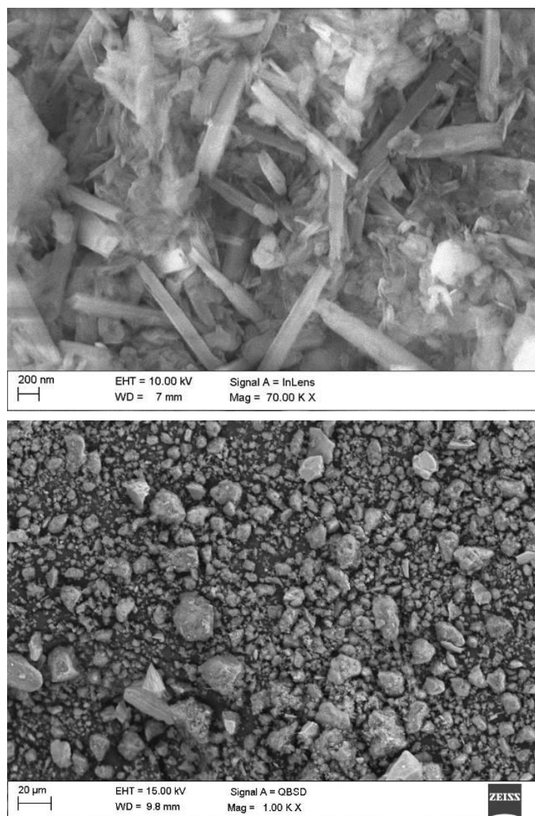
Rys. 4.4 Zdjęcia SEM haloizytu użytego w badaniach
