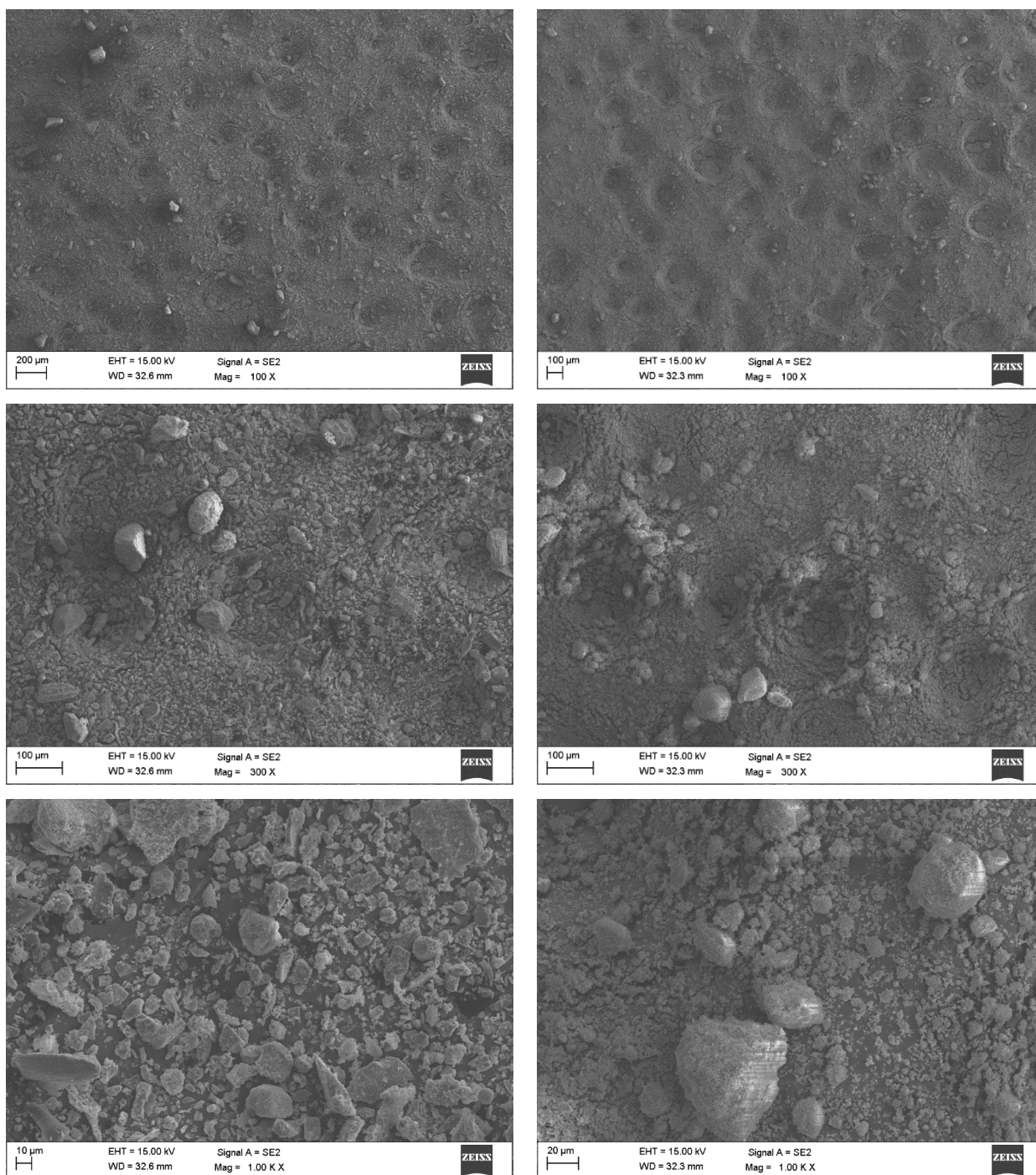
Rys. 10.7 Zdjęcia SEM próbki A2 przed (lewa) i po procesie mielenia (prawa)
