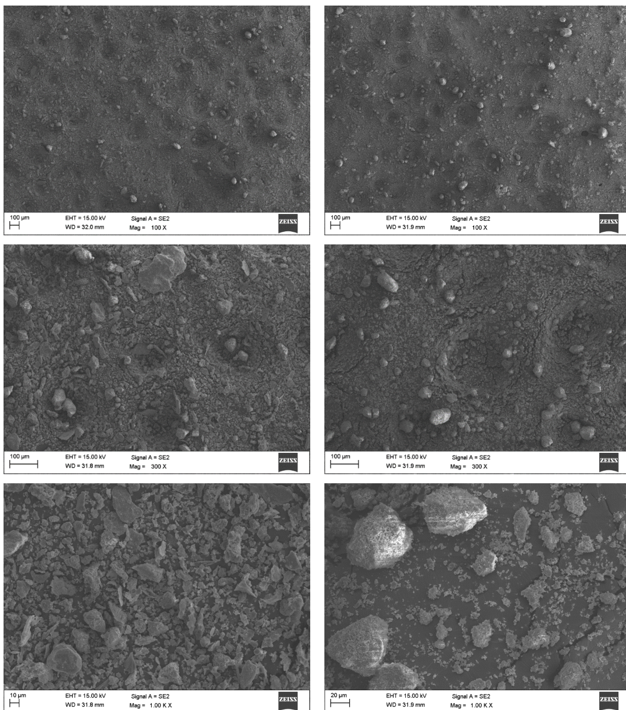
Rys. 10.9 Zdjęcia SEM próbki A4 przed (lewa) i po procesie mielenia (prawa)
