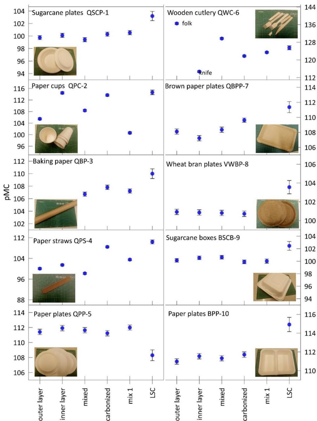
Rys. 8 Porównanie pomiarów stężenia ^{14}\text{C} w DPM metodą LSC i AMS.
