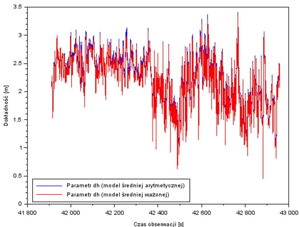
Rys. 9.5. Parametr dh z modelu średniej ważonej i modelu średniej arytmetycznej [opr. wł.]
