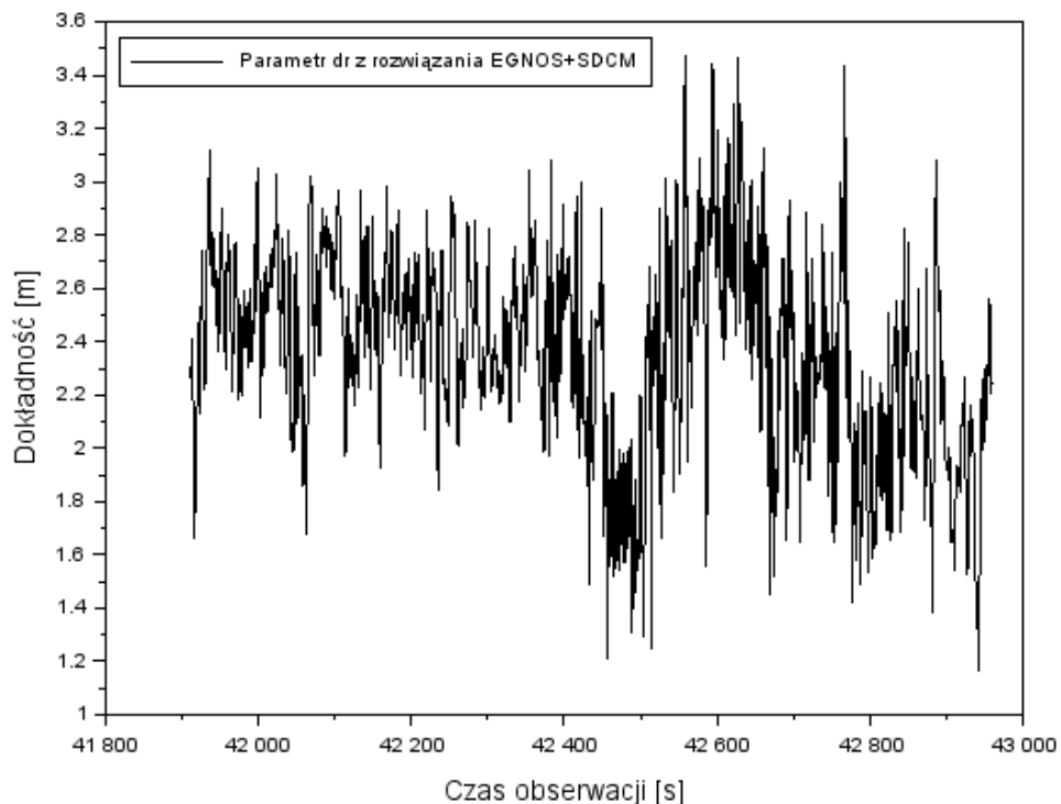
Rys. 8.5. Wektor przesunięcia współrzędnych dr w płaszczyźnie 3D [opr. wł.]
