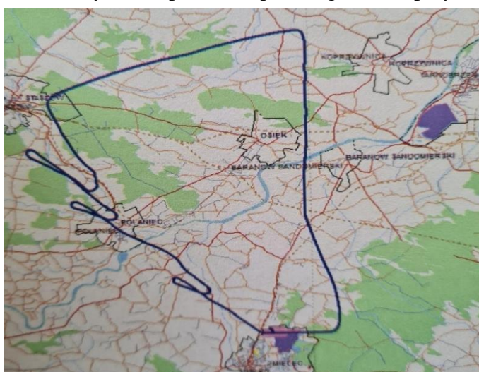
Rys. 7.11. Trajektoria samolotu Cessna dla testu lotniczego nr 7 [24]
