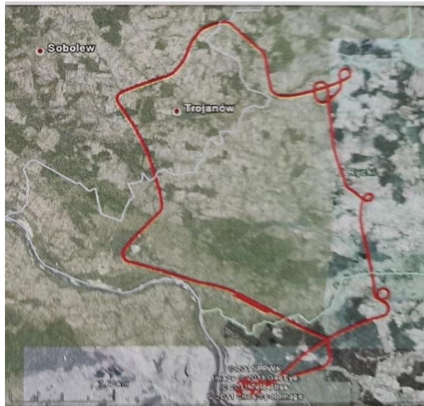
Rys. 7.3. Trajektoria samolotu Cessna dla testu lotniczego nr 3 [21]
