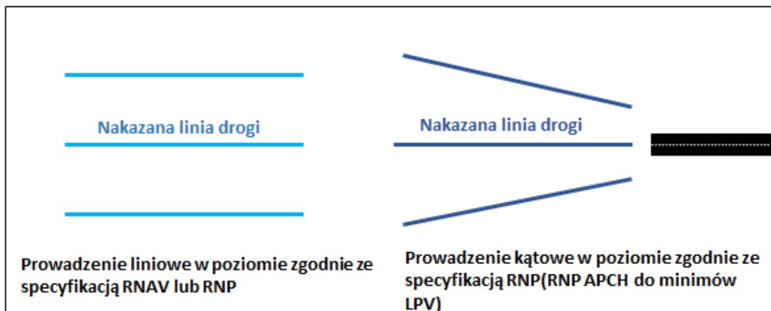
Rys. 3.4. Rodzaje prowadzenia poziomego [opr. wł. na podstawie 88]
