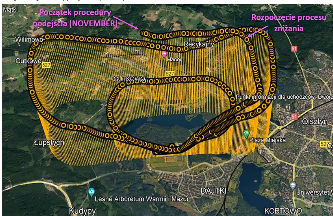
Rys. 7.26. Trajektoria pozioma podejścia do lądowania z rozwiązaniem EGNOS+SDCM [opr. wł.]
