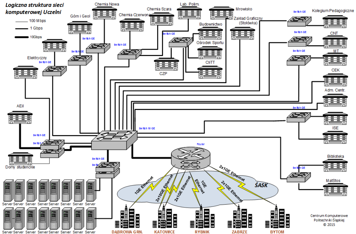
Rysunek 42. Logiczna struktura sieci komputerowej Uczelni
