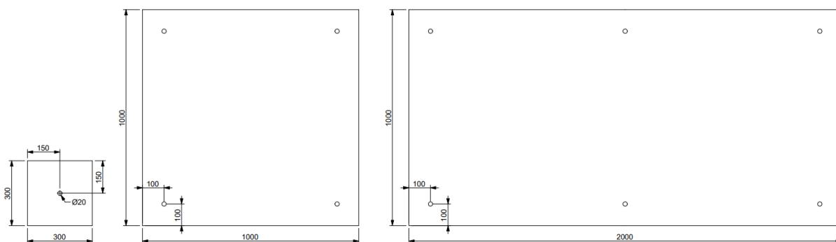
Rys. 1 Rodzaje próbek: 300 mm × 300 mm, 1000 mm × 1000 mm, 1000 mm × 2000 mm.
