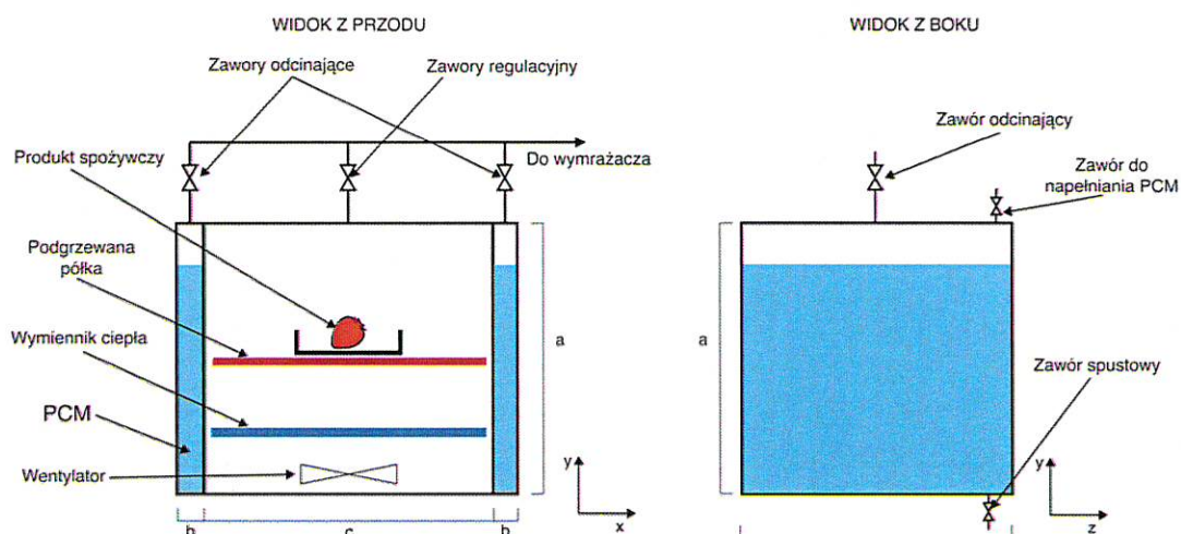
Rys. 2 Schemat komory próżniowej
